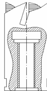
wiertło aparatu do nawiercania PCV
