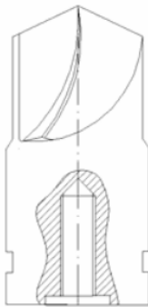
wiertło aparatu do nawiercania ŻL/ST/AC
